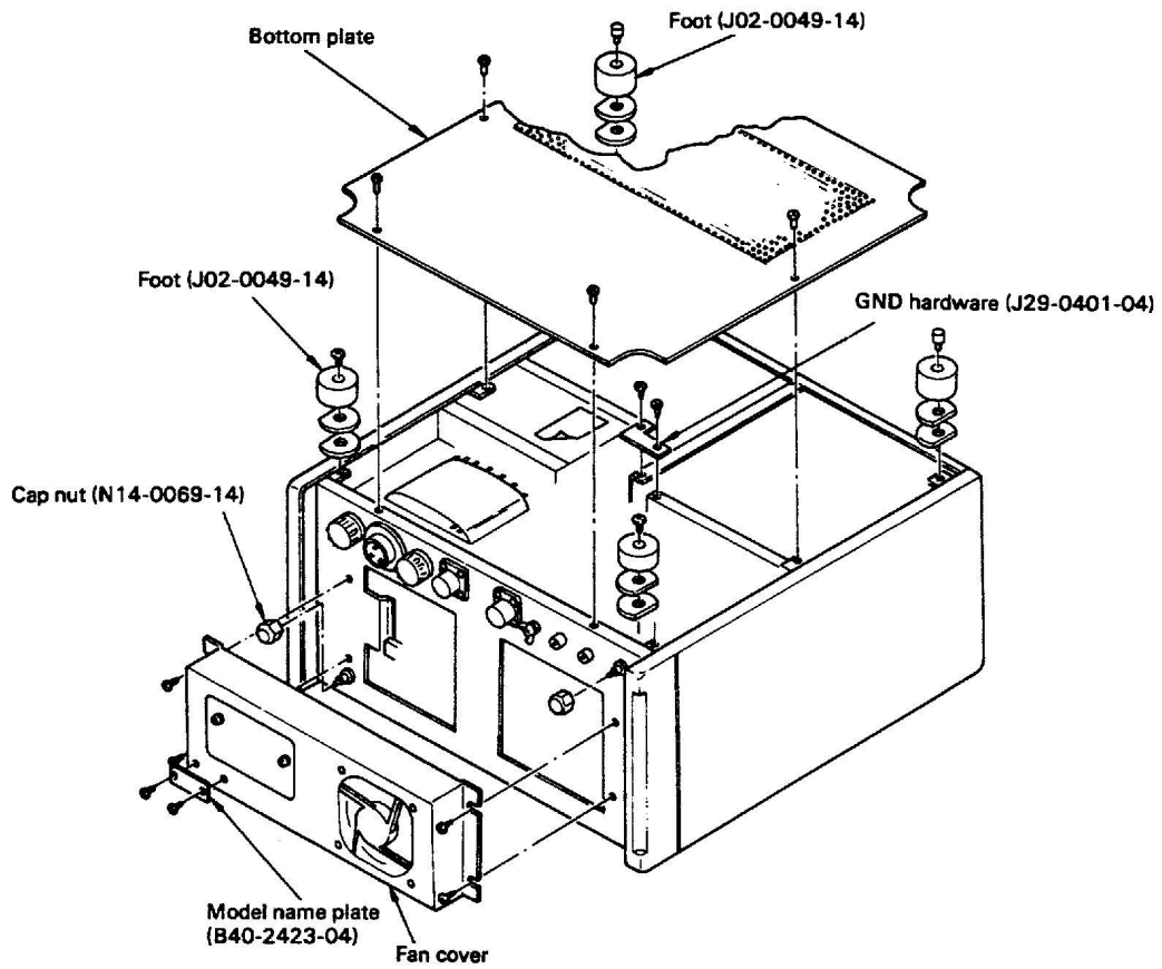
Fig. 6 Subpanel
